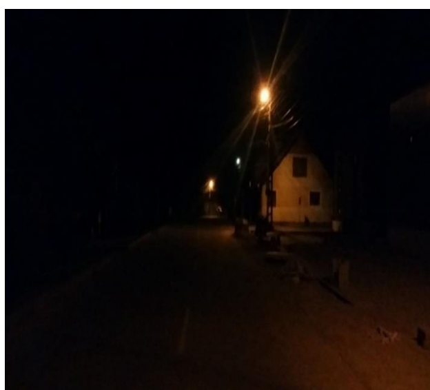
Strada Principala DJ593 clasa M5-Luminanțe insuficiente cca 0,2 cd/m 2
