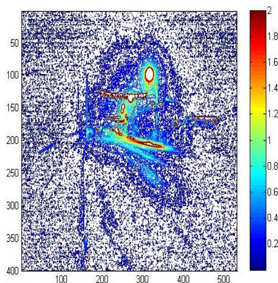
Strada Principala DJ593 clasa M5-Luminanțe insuficiente cca 0,2 cd/m 2
